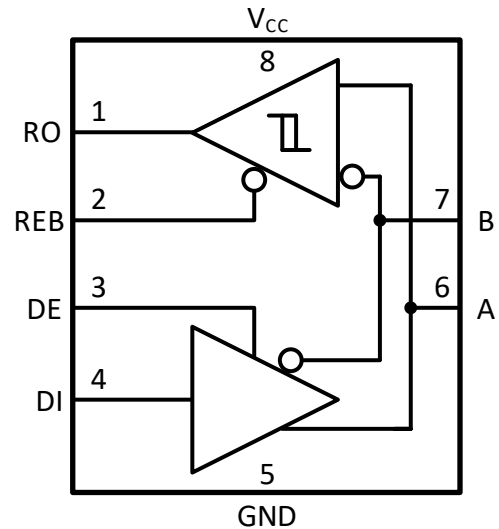
图 3-1 简化原理图
