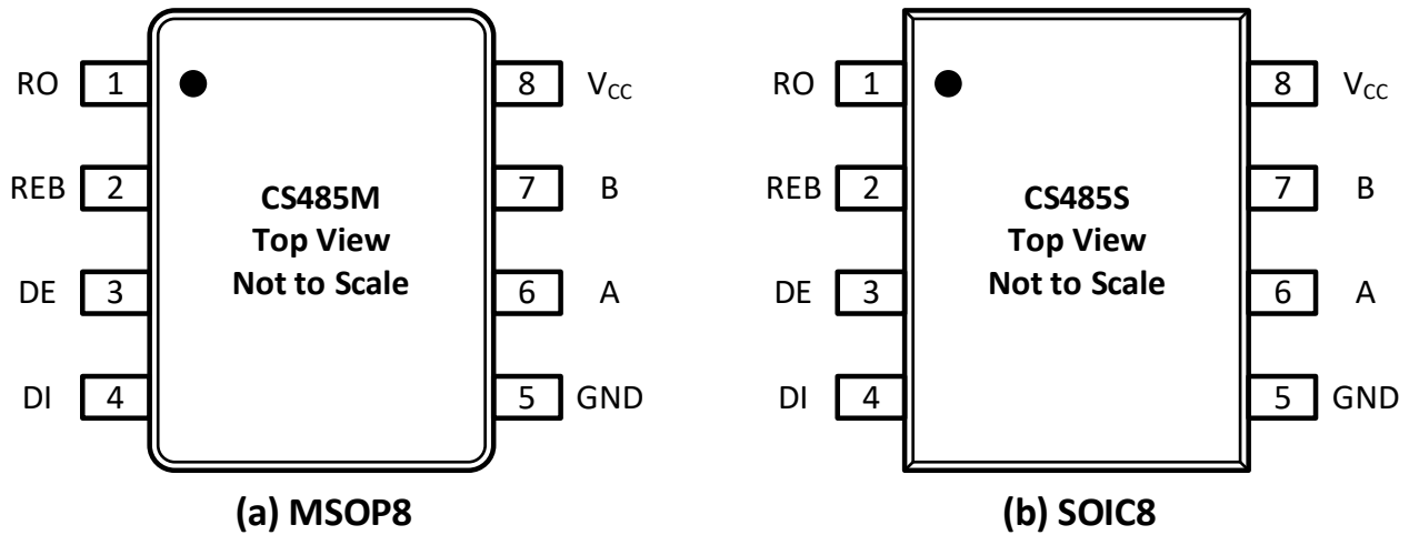
图 6-1 CS485 引脚图：(a) MSOP8；(b) SOIC8
